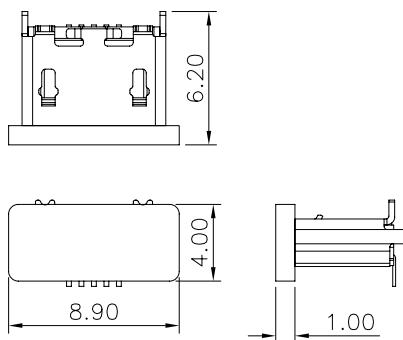
装上CAP尺寸示意图 比例1:2
