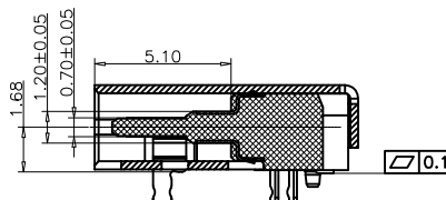
SECTION A-A SCALE 1:1
