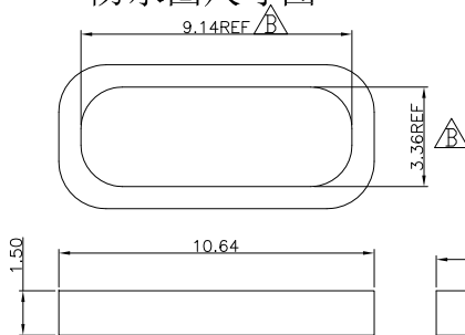
防水圈尺寸图
